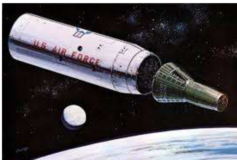
Efter att programmet avslutats, skildes rymdfarkosten Gemini B och laboratoriet åt. Gemini B landade med astronauterna ombord, medan laboratoriet lämnades åt sitt öde runt jorden.
