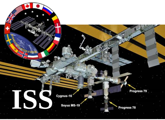
ISS Rymdstation
