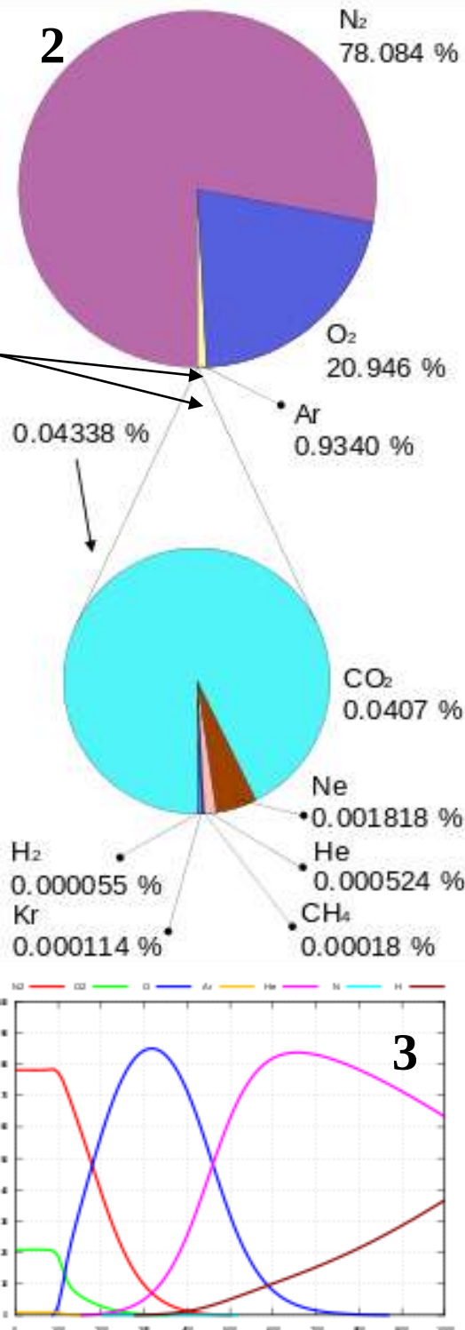
Graf: Kväve N 2 , Syre O 2 , Argon Ar
