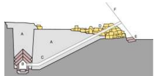
Enligt ritningen liknade Djedefras gravkammare Djoser's, vars gravkammare låg under pyramiden.
