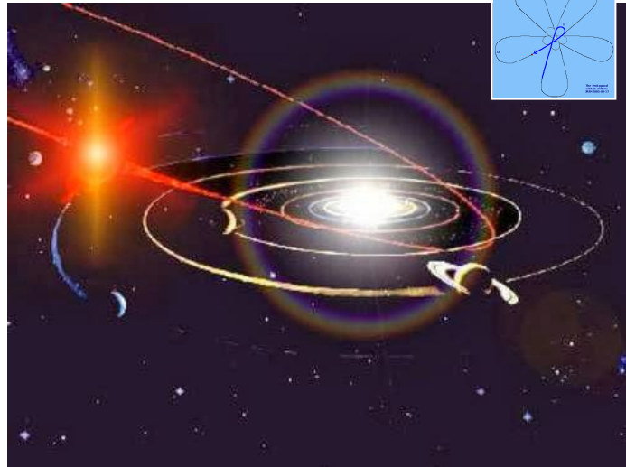
Bilden illustrerar Nemesis bana i vårt solsystem. OBS att Nibiru här illustreras som en stjärna, som rundar solen.
