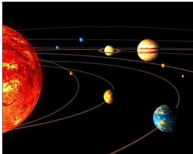
Bilden, illustrerar vårt solsystem med solen i centrum, bl.a. de kretsande planeterna Merkurius, Venus, jorden, Mars, Jupiter, Saturnus, Uranus, Neptunus och Pluto.
