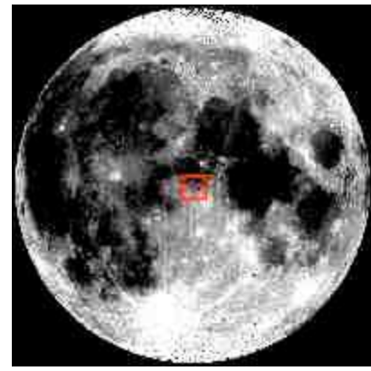
Hyginus Rille.
