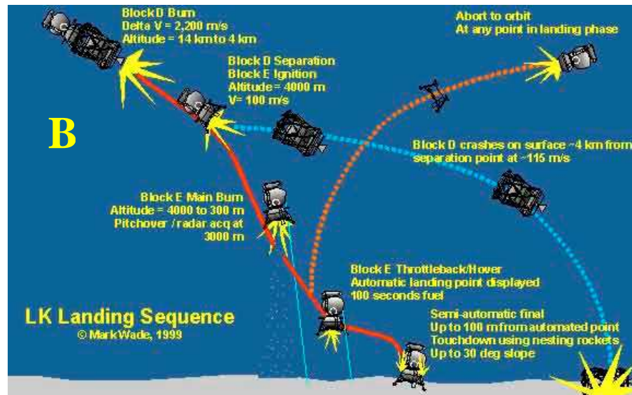
Runt månen
