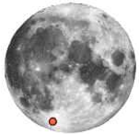
Tycho krater
