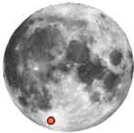
Tycho krater
