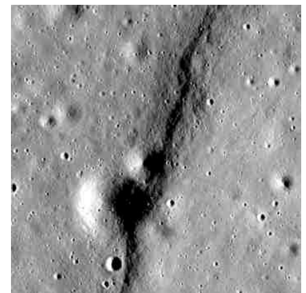
Chang'e 1 störtar....
