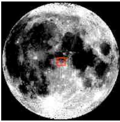
Hyginus Rille.
