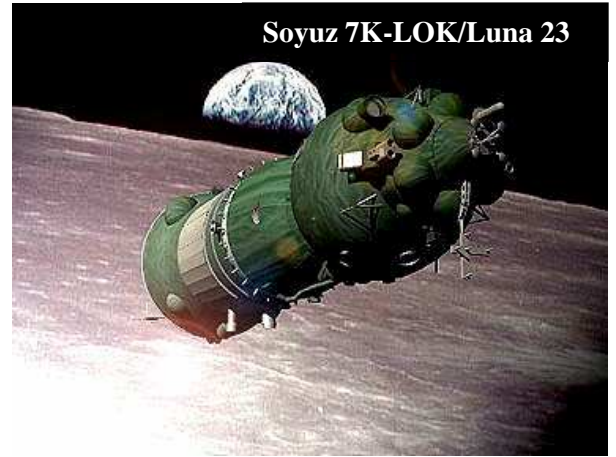
Runt månen
