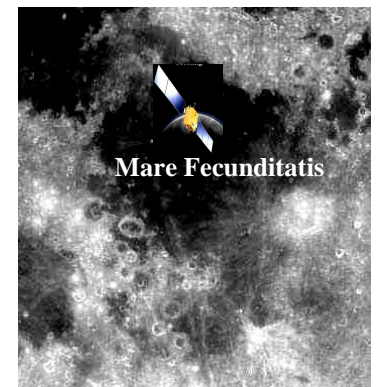
Chang'e 1 störtar....
