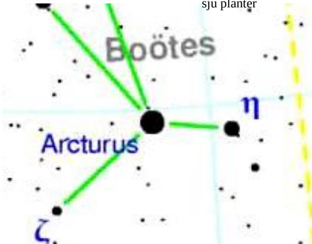
Stjärnbilden Björnvaktaren
