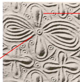
Inannas modell 1 och modell 2 om neutronstjärnan AN:s (Nemesis) pentagonala bana runt solen. Till höger om hennes modeller ser vi dagens Nemesis pentagonala bana runt solen.
