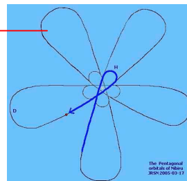
Inannas modell 1 och modell 2 om neutronstjärnan AN:s (Nemesis) pentagonala bana runt solen. Till höger om hennes modeller ser vi dagens Nemesis pentagonala bana runt solen.
