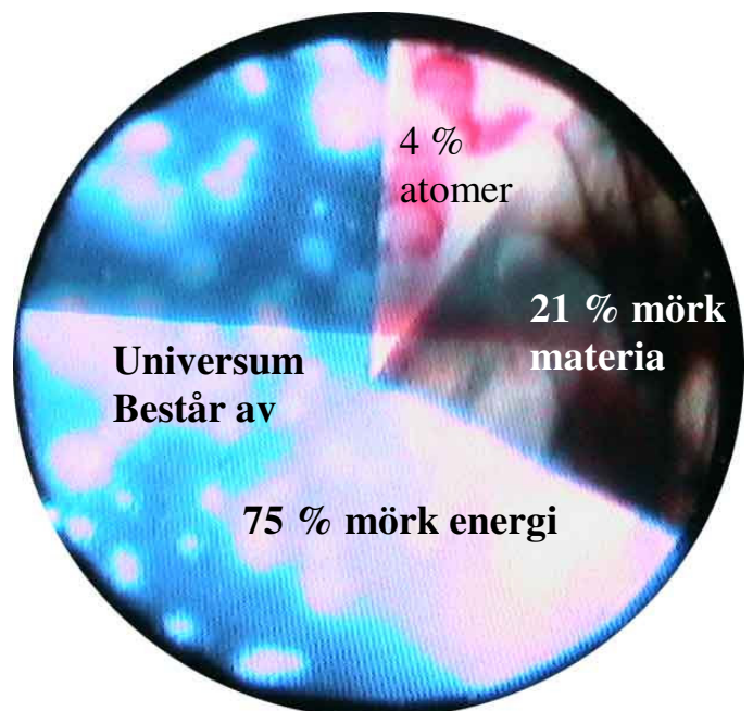
Kosmologiska standardmodellen
